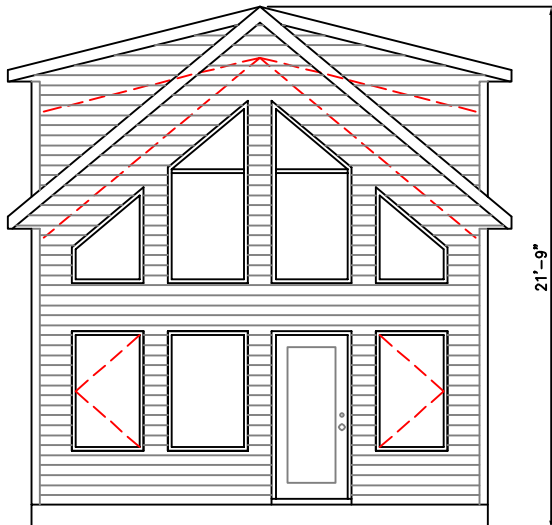
FRONT ELEVATION SCALE: 1/8"=1'-0"
